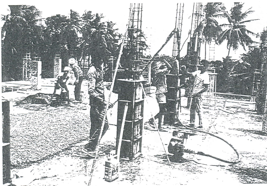
P.T. Parru, storten kolommen 2e verdieping kindertehuis
