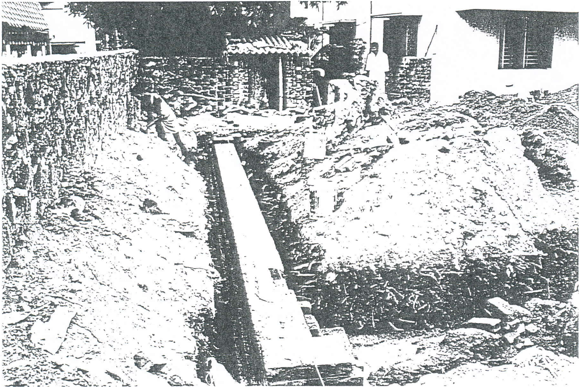
Madras St. Louis Convent, fundatiewerken naai- en typeschool
